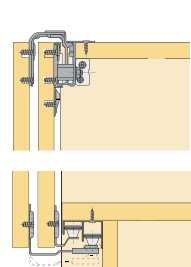
Система розсувних дверей TopLine L
